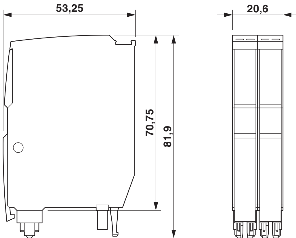
Rysunek wymiarowy
