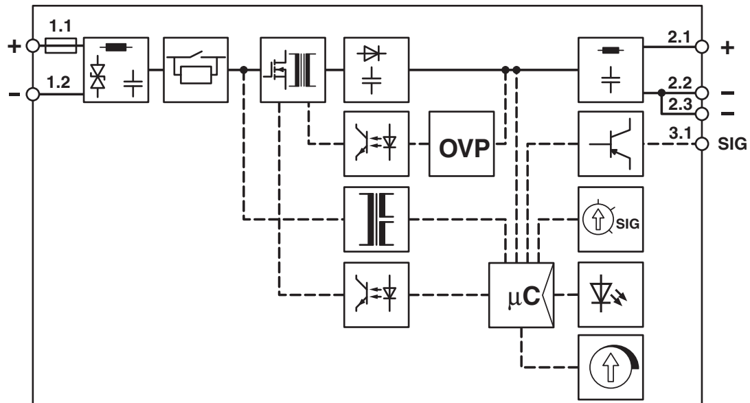
Schemat blokowy
