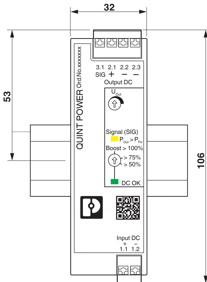
Rysunek wymiarowy
